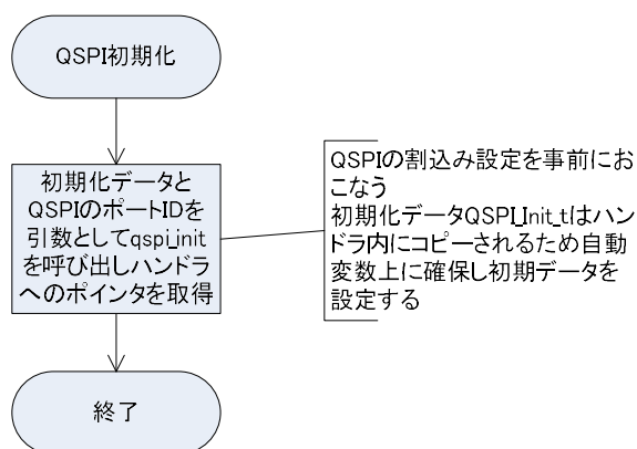
図 4.2.6.3.1 QSPI 初期化
