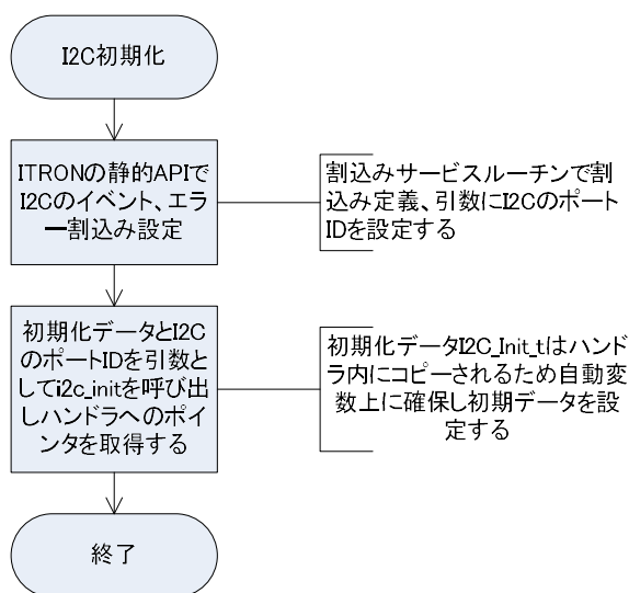
図 4.2.2.3.1 初期化フローチャート
