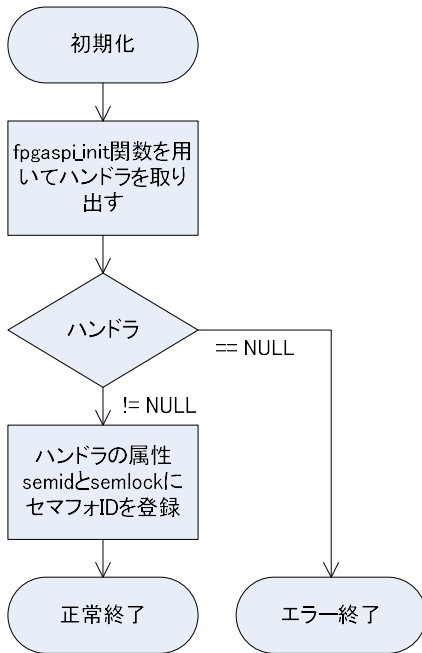
図 4.3.4.3.1 初期化
