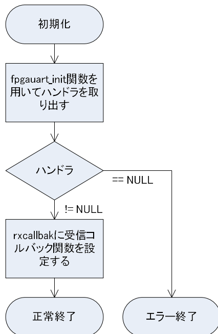
図 4.3.3.3.1 初期化
