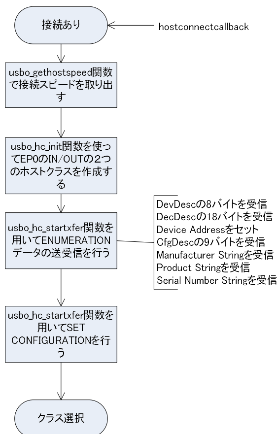
図 4.2.5.3.2 接続処理
