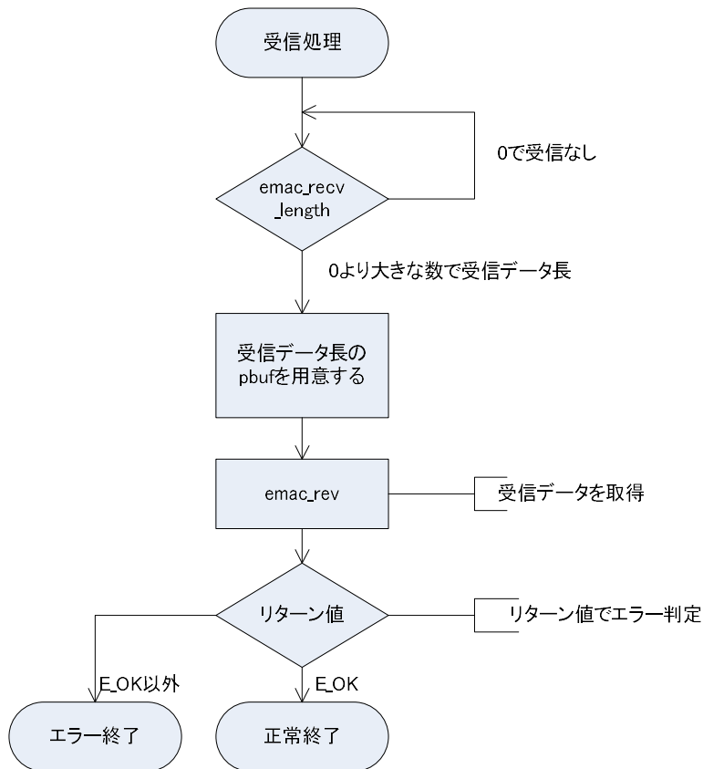
図 4.2.7.3.3 EMAC 受信
