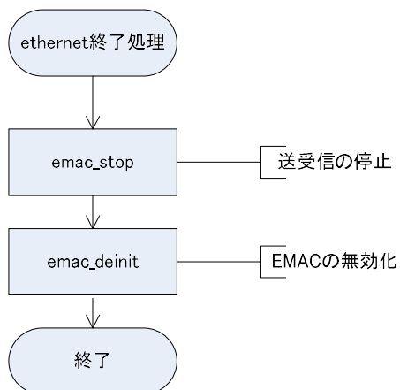
図 4.2.7.3.4 EMAC 終了処理
