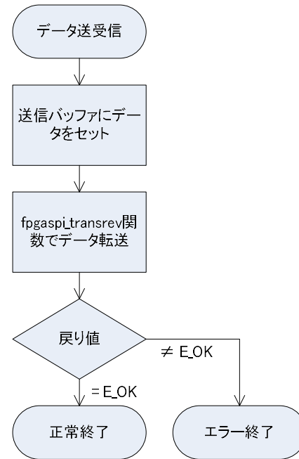
図 4.3.4.3.2 データ転送
