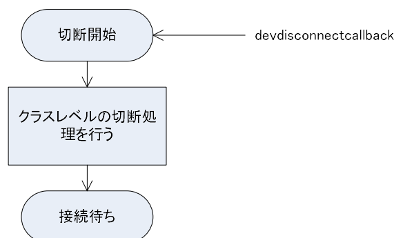
図 4.2.5.3.6 USB デバイスの切断
