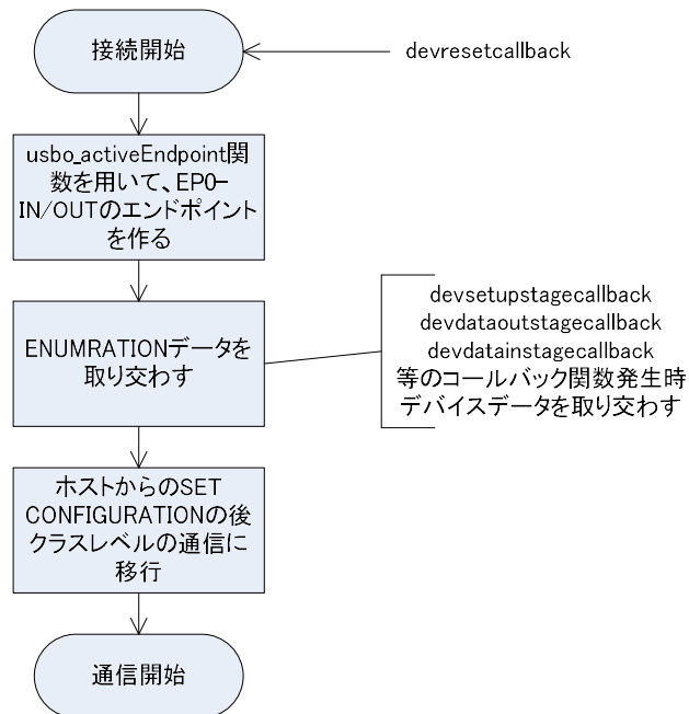
図 4.2.5.3.5 USB デバイスの接続
